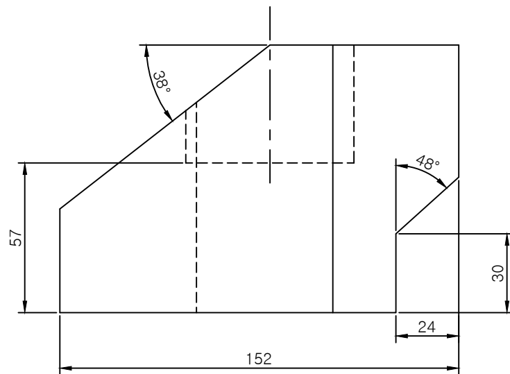
정면도 축척 1/2
