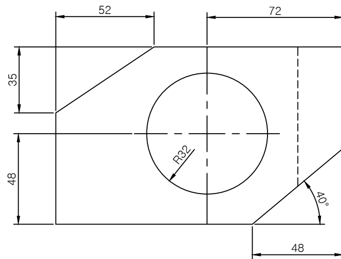
평면도 축척 1/2
